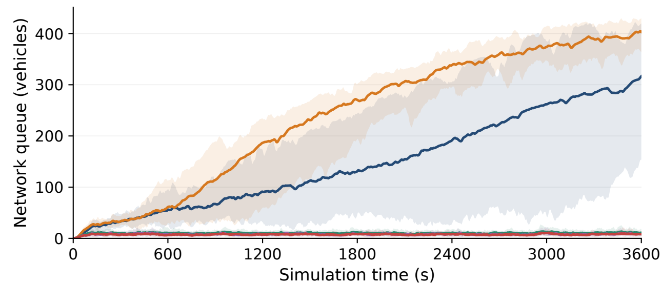
PPO
