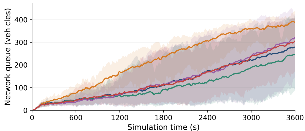
IQLL
